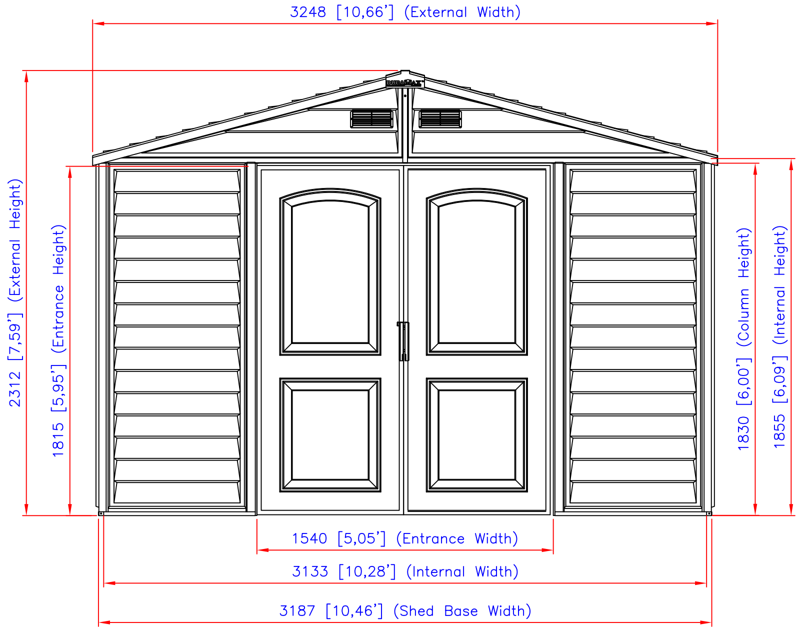
Elevation
