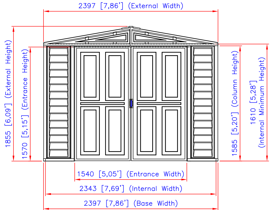
Elevation
